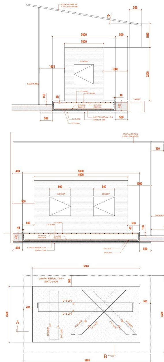
Gambar 4. Desain Pondasi Genset RSI AY
