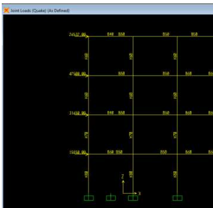
Gambar 9. Beban Gempa Portal melintang
